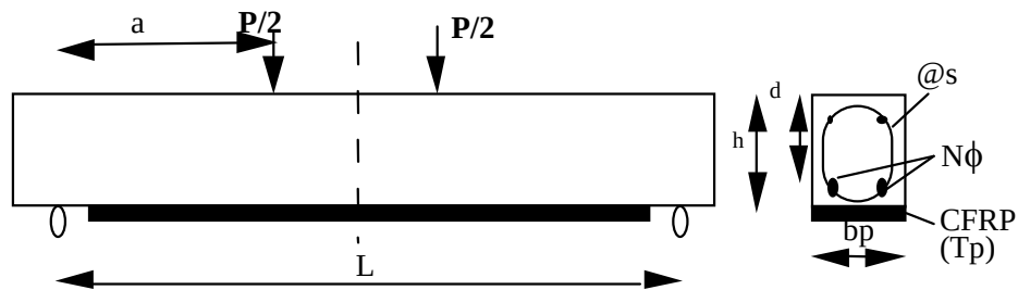
شکل ۷- تیر بتنی تقویت شده
