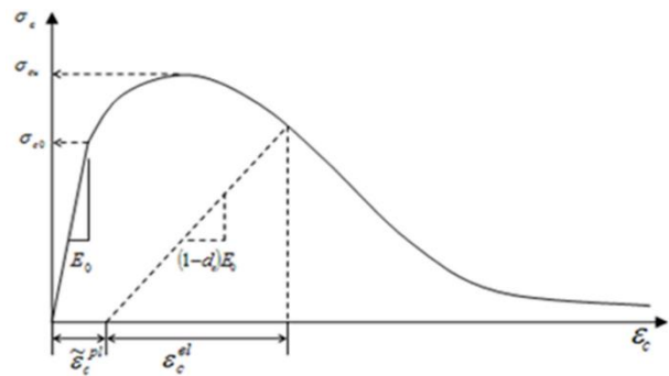
شکل ۵- منحنی تنش - کرنش فشاری مدل خسارت پلاستیک [۱۰]
