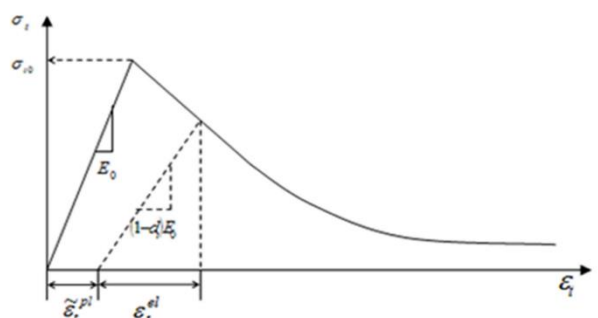
شکل ۶- نمودار تنش - کرنش کششی مدل خسارت پلاستیک [۱۰]
