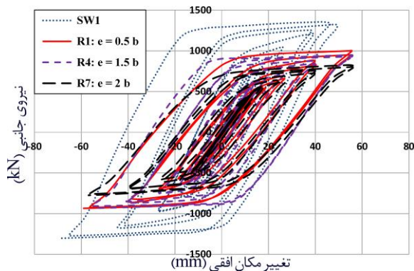
شکل ۱۸- منحنی هیسترسس نمونه‌های SW1، R1، R4 و R7
