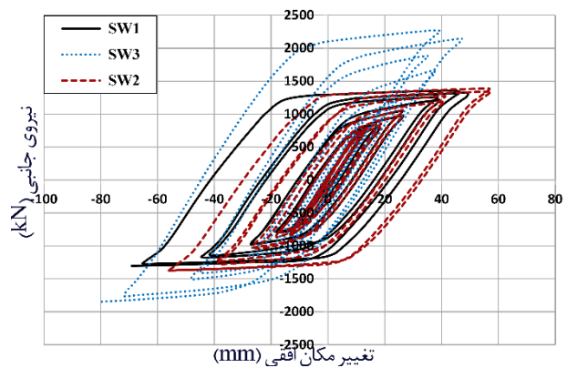
شکل ۱۳- منحنی هیسترسیز نمونه‌های SW1، SW2 و SW3
