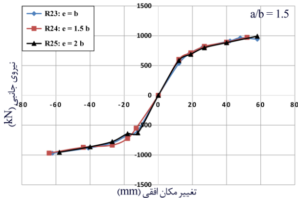
شکل ۳۰- پوش هیسترسیز نمونه های R23، R24 و R25
