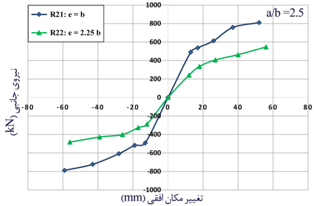
شکل ۲۹- منحنی پوش هیسترسیز نمونه های R21 و R22
