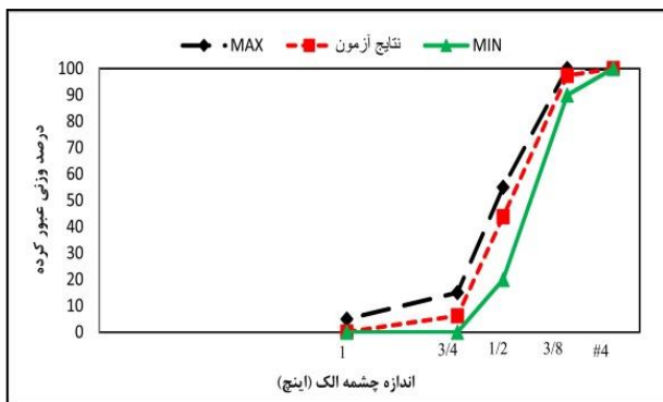
شکل ۴- منحنی دانہ بندی شن
