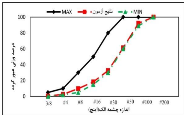
شکل ۵- منحنی دانه بندی ماسه
