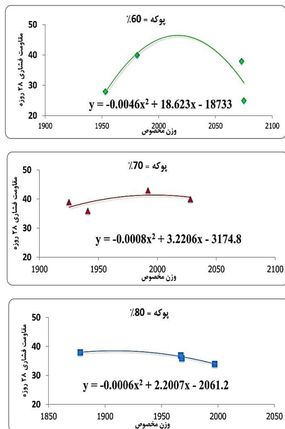
شکل ۲- تغییرات مقاومت فشاری بر حسب تغییرات وزن مخصوص، به ازای مقادیر ثابت پوکه
