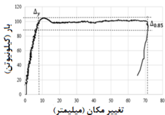
شکل ۲۰- شکل پذیری نمونه OR-10T
