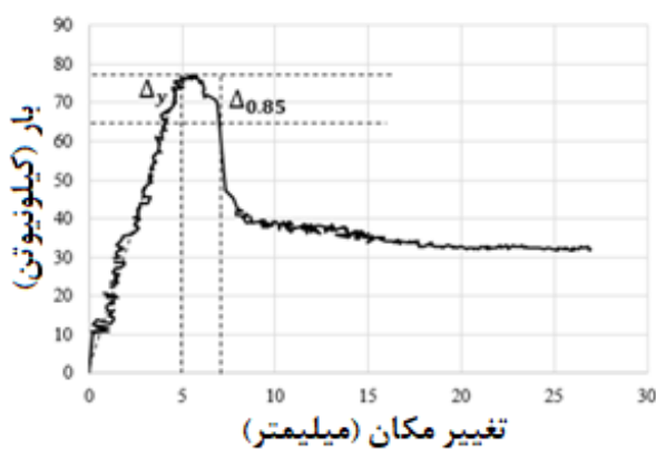
شکل ۱۵- شکل پذیری نمونه 50R-WT
