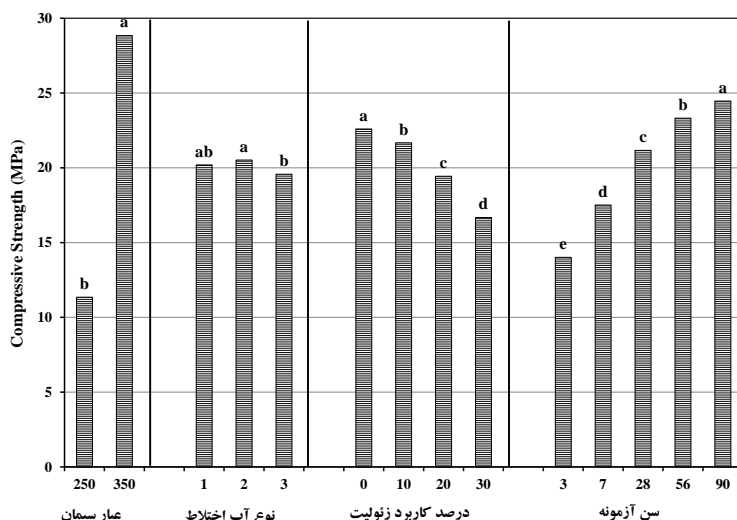
شکل ۲- اثر ساده عیار سیمان، نوع آب، درصد کاربرد ژئولیت و سن آزمون بر مقاومت فشاری آزمون‌های بتنی
