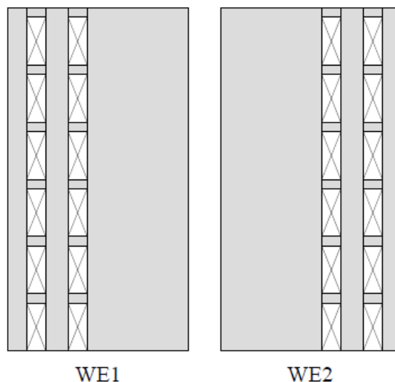
شکل ۱۵- نمونه‌های طراحی شده دارای دو ردیف گشودگی به صورت غیر متقارن
