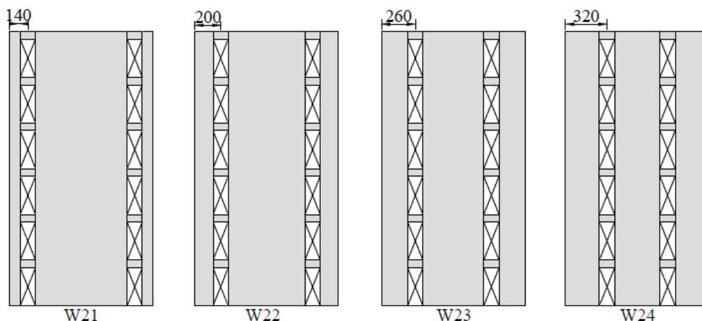
شکل ۱۰- نمونه‌های طراحی شده دارای دو ردیف گشودگی
