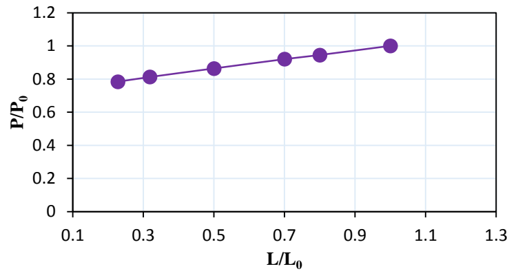
شکل ۱۲- تأثیر موقعیت گشودگی بر روی ظرفیت برشی دیوارهای بتن مسلح
