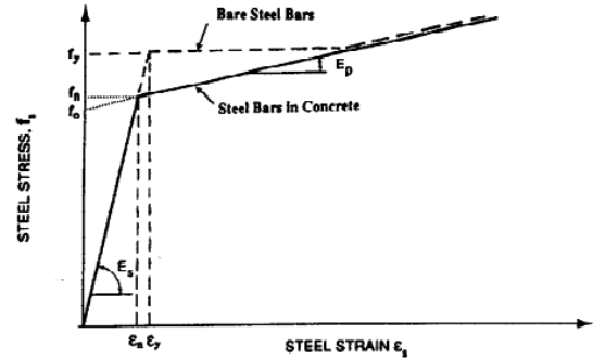
شکل ۶- مدل رفتاری بلاری [۱۲]
